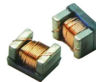
铁氧体 (Ferrite)
